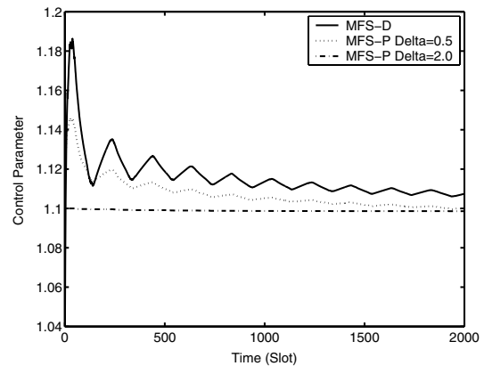
Fig. 2. MFS-D and MFS-P Control Parameter Update
